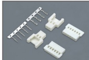
20012(2.00mm) P34
