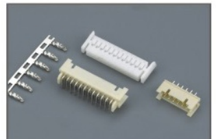
PHD-S(2.00mm) P32
