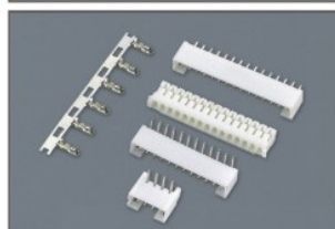
PH(2.00mm) P23
