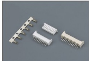
51021(1.25mm) P12
